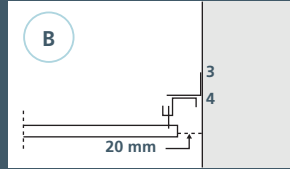
Veggprofil, justerbar
